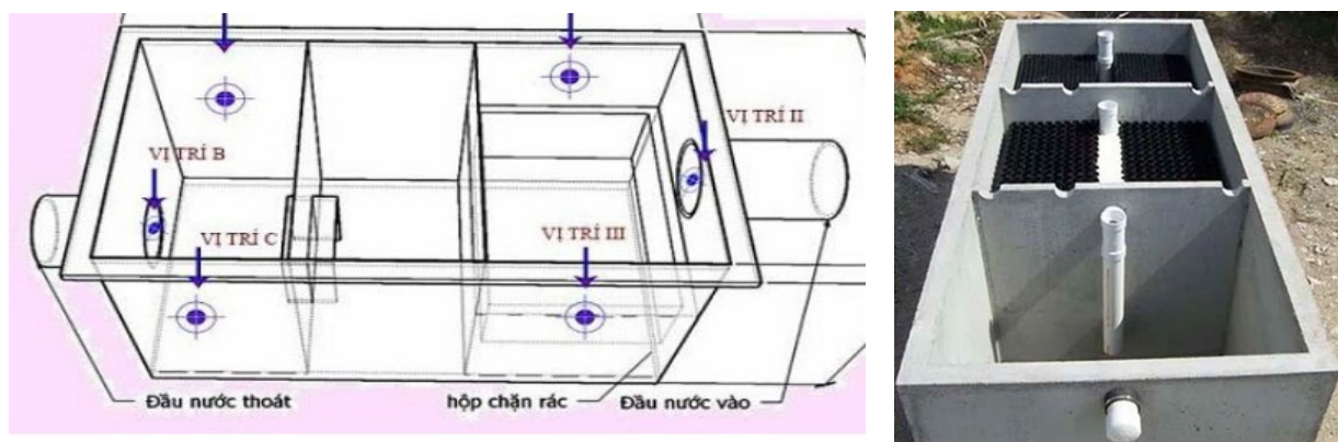
Hình 3.3. Cấu tạo bể tách dầu tại cửa hàng
